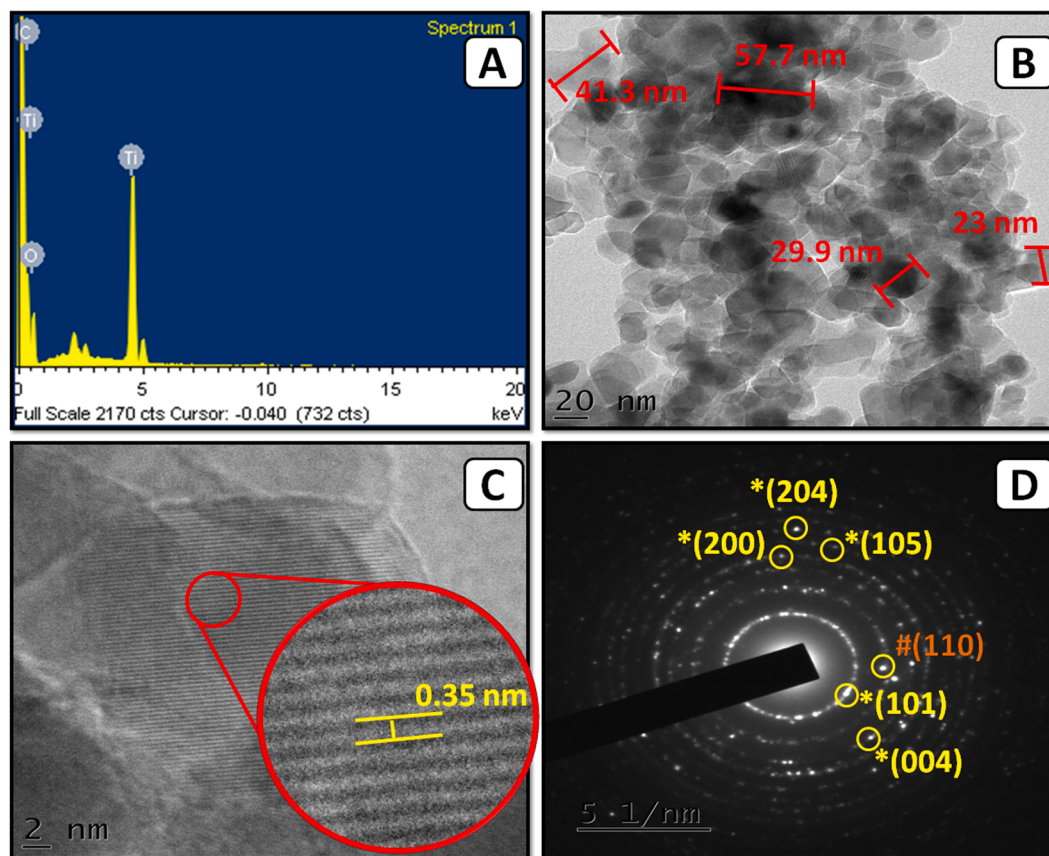
Fig. 2. EDX (A), HRTEM image (B&C) and SAED pattern (D) of nano \text{TiO}_2 -10% PANI composite.
