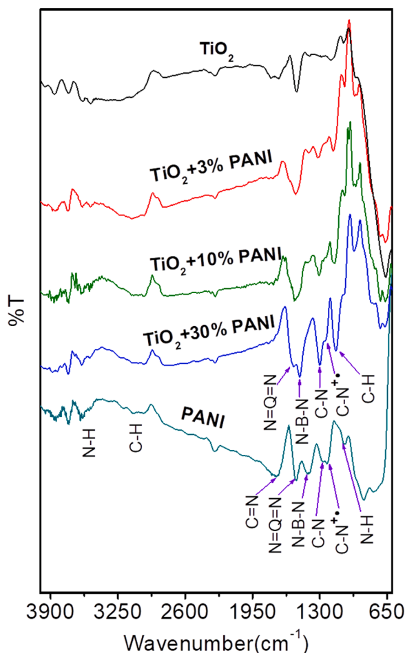
Fig. 3. FTIR spectra of TiO 2 , PANI and TiO 2 -PANI composites,
